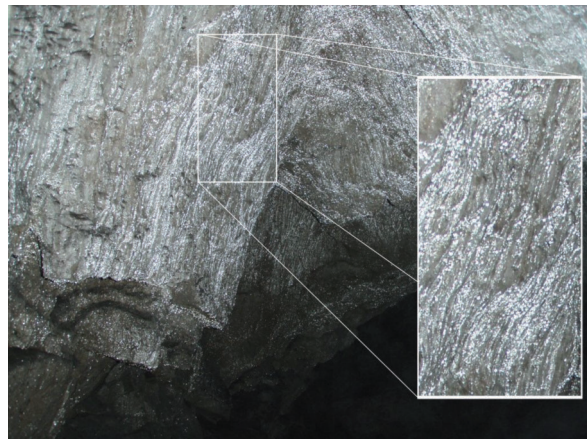
Fig. 8: Condensation in Treeumphant passage near Crowning Glory. Streaks detailed in inset are interpreted in the text as rivulets down which condensate slowly flows. Kondensation im Treeumphant Gang nahe Crowning Glory. Die Fäden im Detailbild werden als kleine Rinnsale interpretiert, entlang denen das Kondenswasser langsam nach unten fließt.
